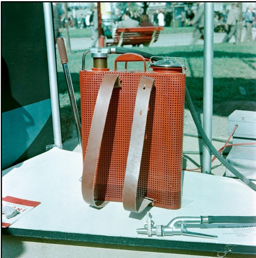
Stříkačka na záda typ SZ - 20
