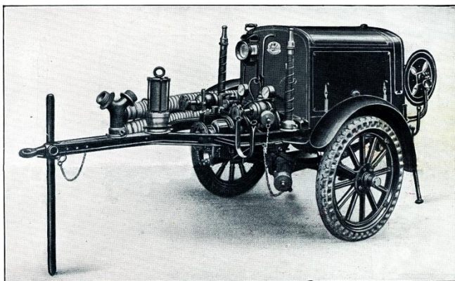
Dvojkolesová motorová stříkačka s elastickými komôrkovými obručami gumenými. — Obr. č. 7.
