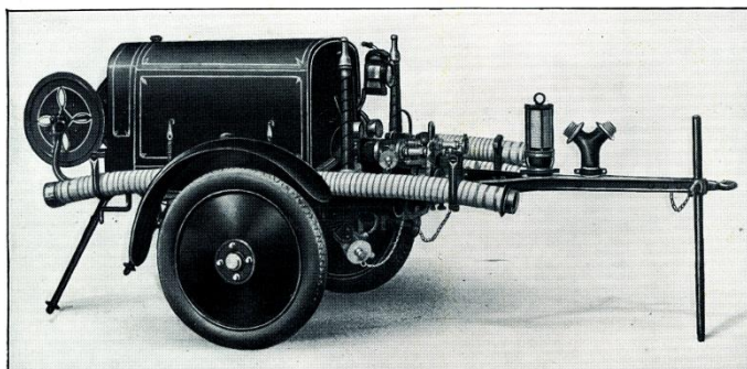
Dvojkolesová motorová stříkačka na diskových kolech s pneumatikami. — Obr. č. 6.
