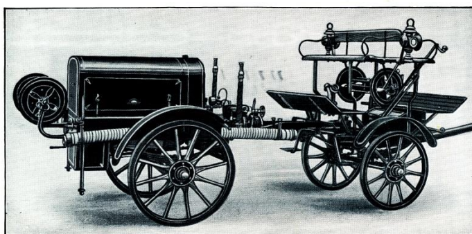
Dvojkolesová motorová stříkačka na kolech lafetových s predným vozom pre dopravu mužstva. — Obr. č. 8.
